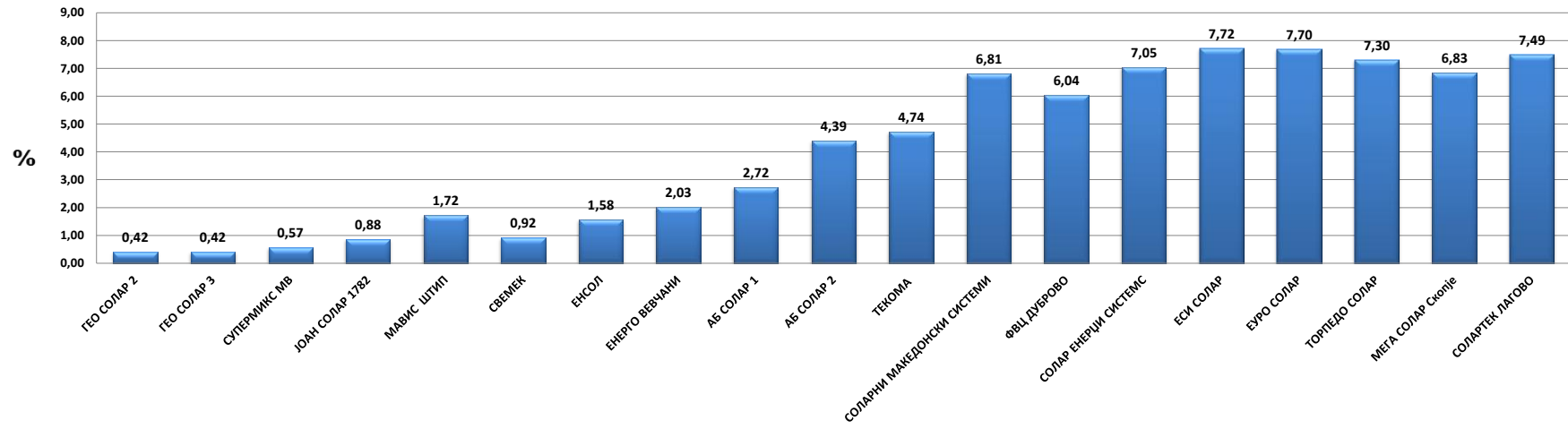
Произведена предадена електрична енергија од ППЕЕ - Фотоволтаични системи >50 за период - февруари 2015 година
